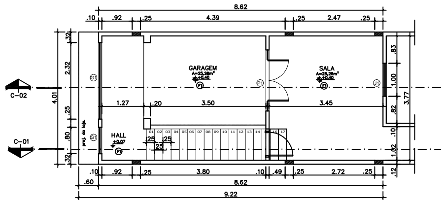
PLANTA BAIXA – EXISTENTE escala.....1:50
