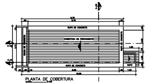
PLANTA DE COBERTURA escala.....1:50
