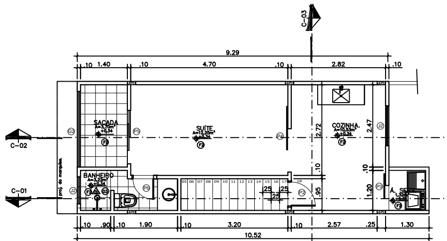
PLANTA PAV. SUPERIOR escala.....1:50
